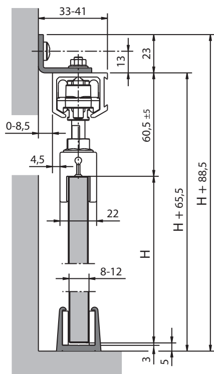
Einbausituation Basic 80 Glas Wandmontage
