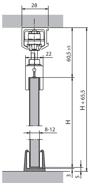
Einbausituation Basic 80 Glas Deckenmontage
