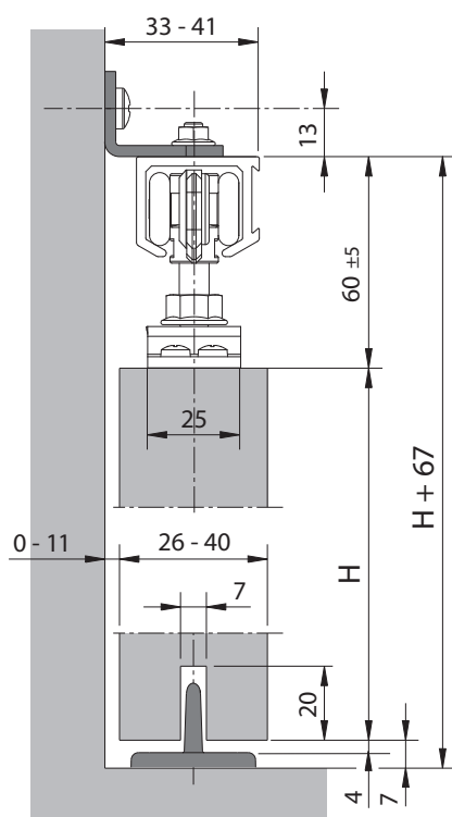
Einbausituation Basic 80 Holz Wandmontage
