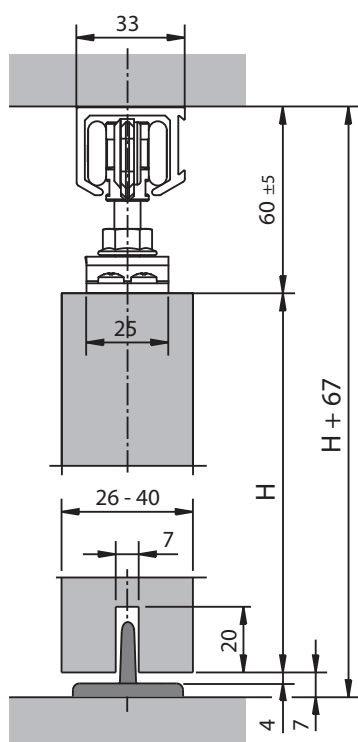
Einbausituation Basic 80 Holz Deckenmontage
